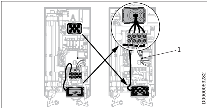
1 電纜佈線
