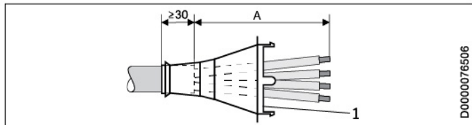
1 電纜扣環
